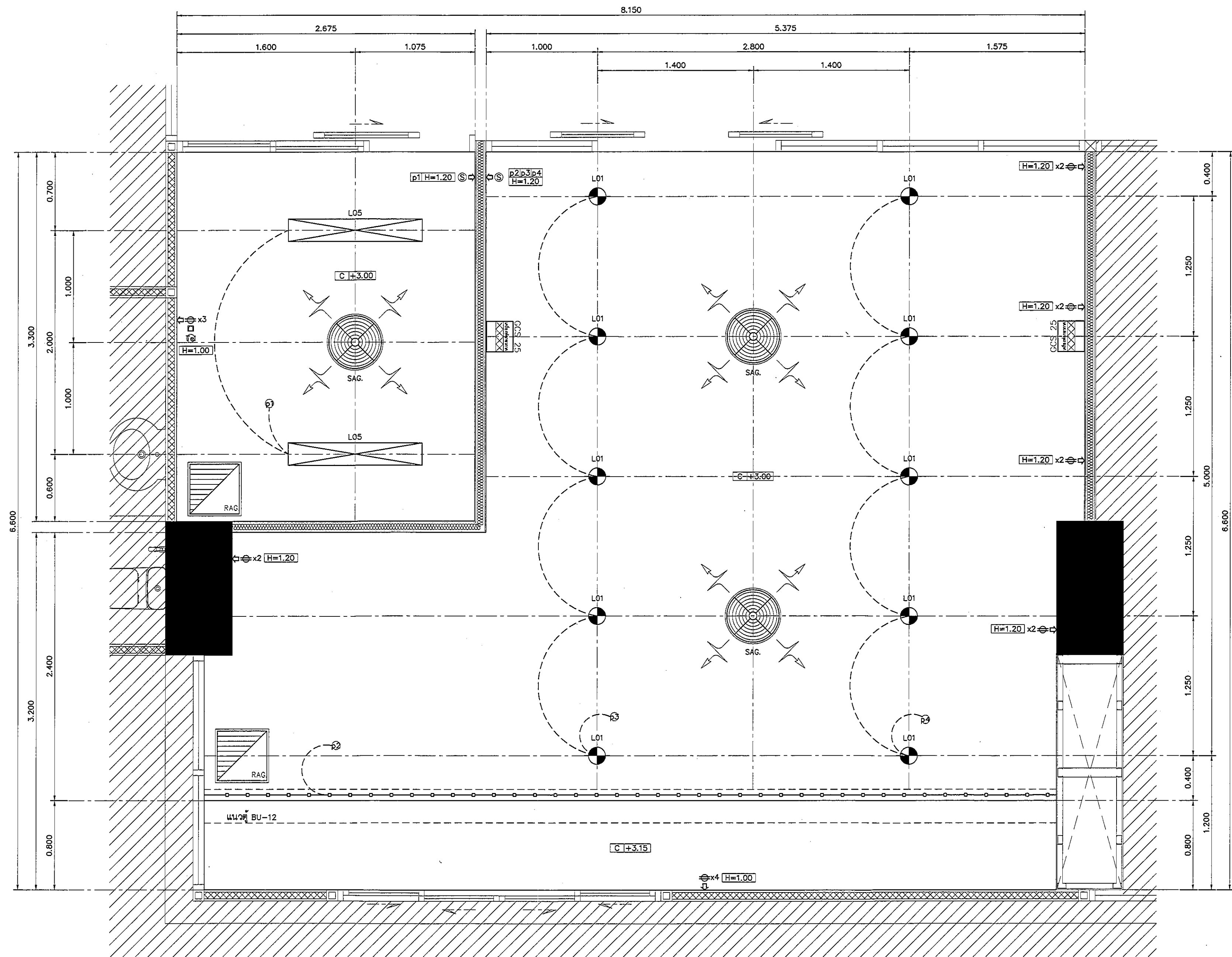
แปลนฝ้าเพดานและงานระบบ ห้องผู้ป่วย/ห้องให้นมบุตร มาตราส่วน 1:25
