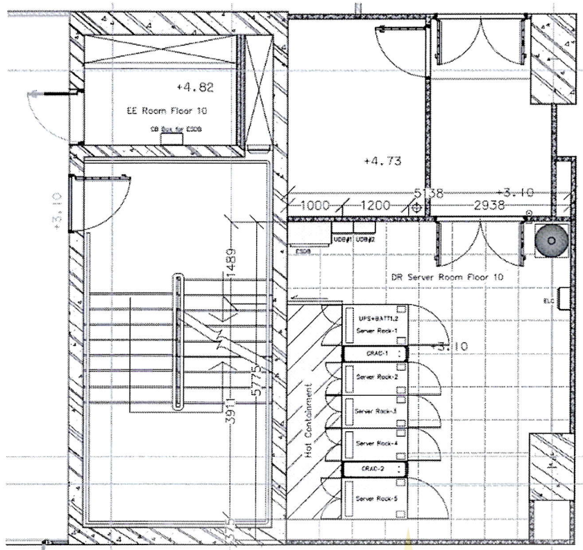
แบบห้องศูนย์คอมพิวเตอร์สำรอง (DR Site) ใหม่
