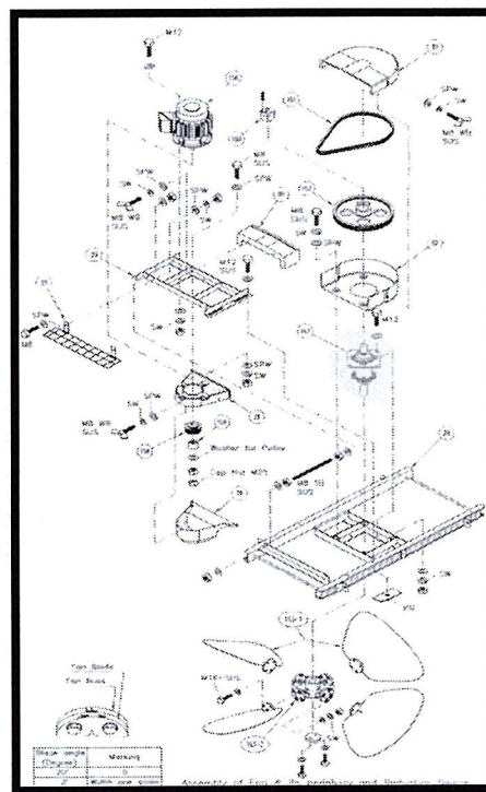
หมายเลข 4 ชุดกล่องลูกปืนใบพัด
